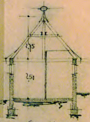
Schnitt a-b
